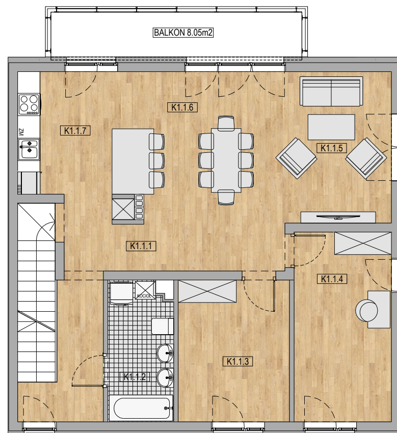
RZUT 1 PIĘTRO
